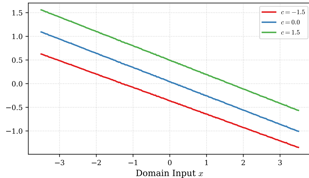
(d) Linear: Variasi Titik Tumpu c
