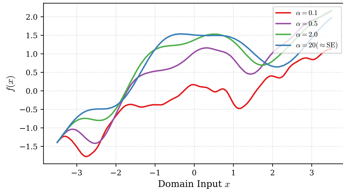
(c) RQ: Variasi \alpha (Multiskala)
